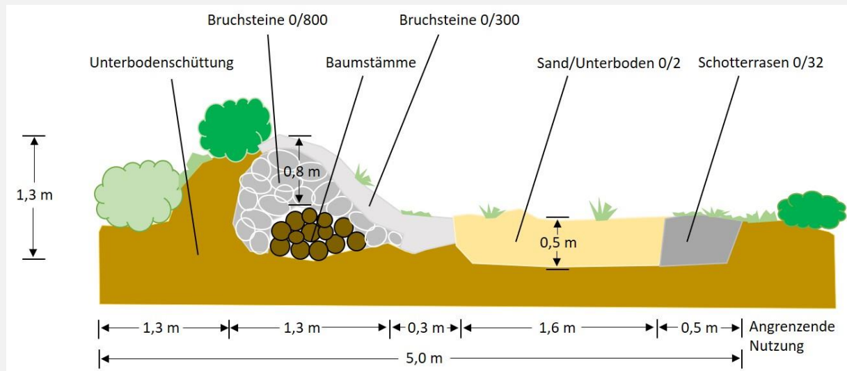
Abb. 12: Schematischer Aufbau eines Steinriegelkomplexes mit Winterquartier, Verwallung und integriertem Eiablagesubstrat. Als Winterquartier dienen frostfrei eingebaute Tothholzelemente.
